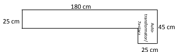
Rys. 1. Widok „z góry” zespołu systemu zasilania (3 szt.)
