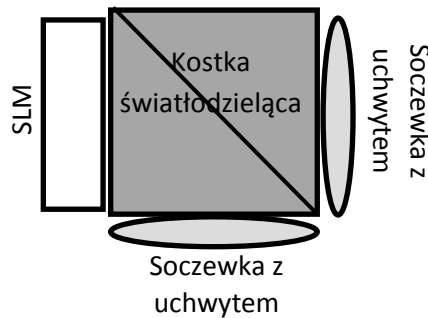
Rysunek 1. Konfiguracja montażu układu przestrzennego modulatora światła (SLM) wraz z kostką światłodzielnyczą i dwiema soczewkami - widok od góry.
