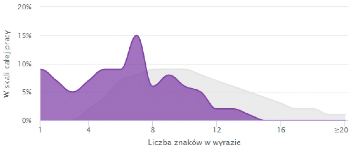
Rozkład długości wyrazów
