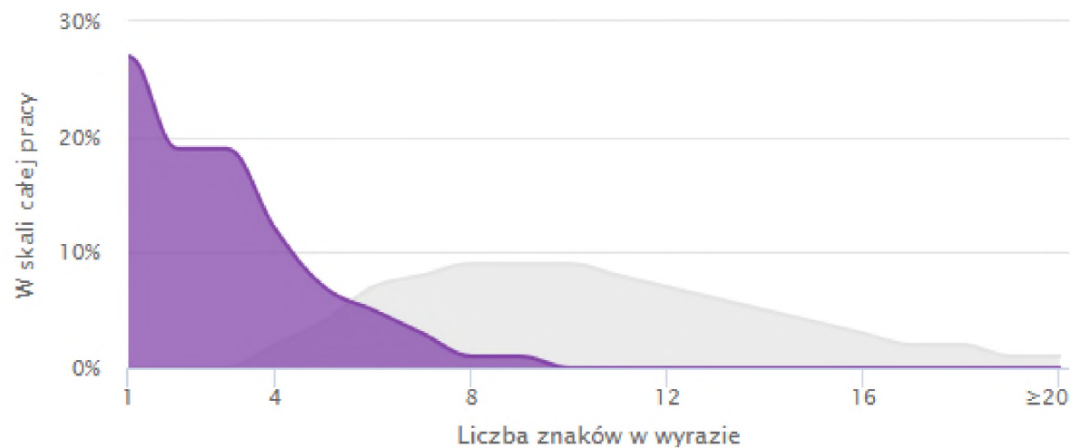
Rozkład długości wyrazów
