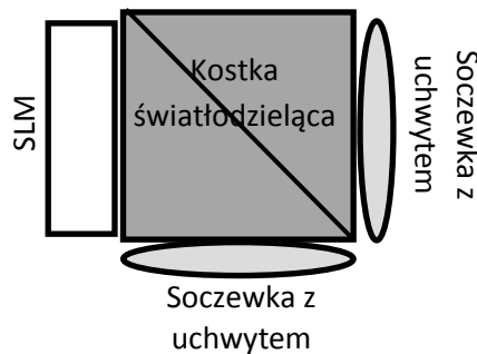
Rysunek 1. Konfiguracja montażu układu przestrzennego modulatora światła (SLM) wraz z kostką światłodzielną i dwoma soczewkami - widok od góry.
