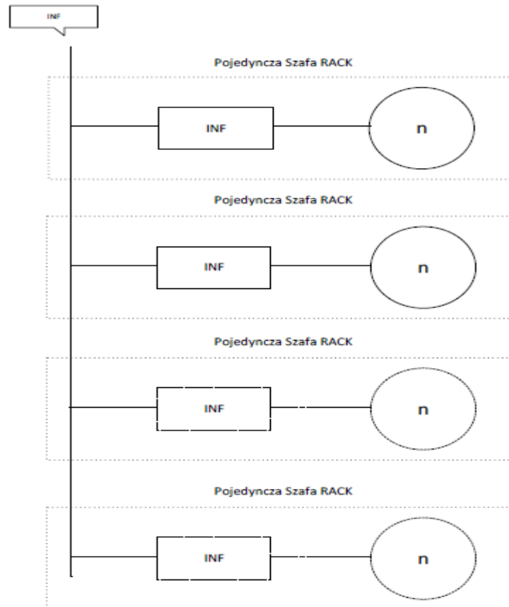
Schemat logiczny połączeń INFINIBAND pomiędzy Szafami RACK
