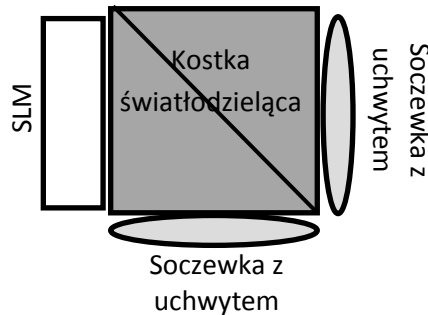
Rysunek 1. Konfiguracja montażu układu przestrzennego modulatora światła (SLM) wraz z kostką światłodziącą i dwiema soczewkami - widok od góry.
