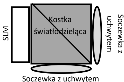
Rysunek 1. Konfiguracja montażu układu przestrzennego modulatora światła (SLM) wraz z kostką światłodzielną i dwoma soczewkami - widok od góry.
